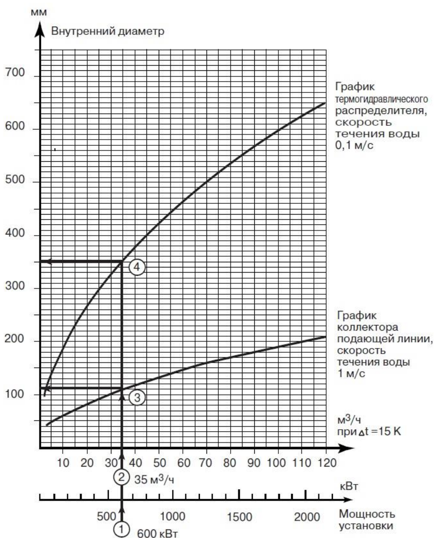
Рисунок 5. График для определения внутреннего диаметра коллекторов
